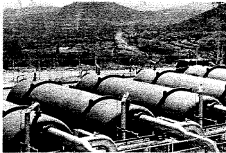
EL SISTEMA de potencia comprende dos grandes plantas de bombeo y 122 kilómetros de ductos, lleva a la presa de almacenamiento 400 mil metros cúbicos.
