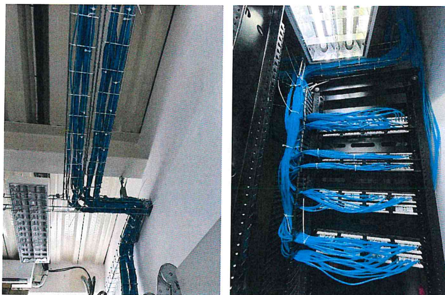
Instalación de cableado estructurado de red de voz y datos
