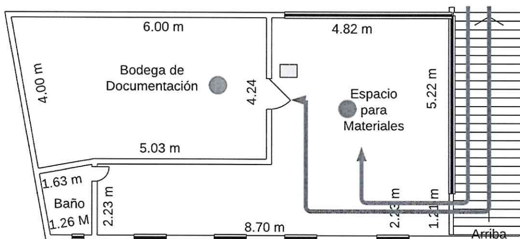
Planta alta
